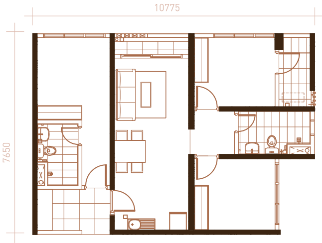
TYPE A3 - 844 sq ft
